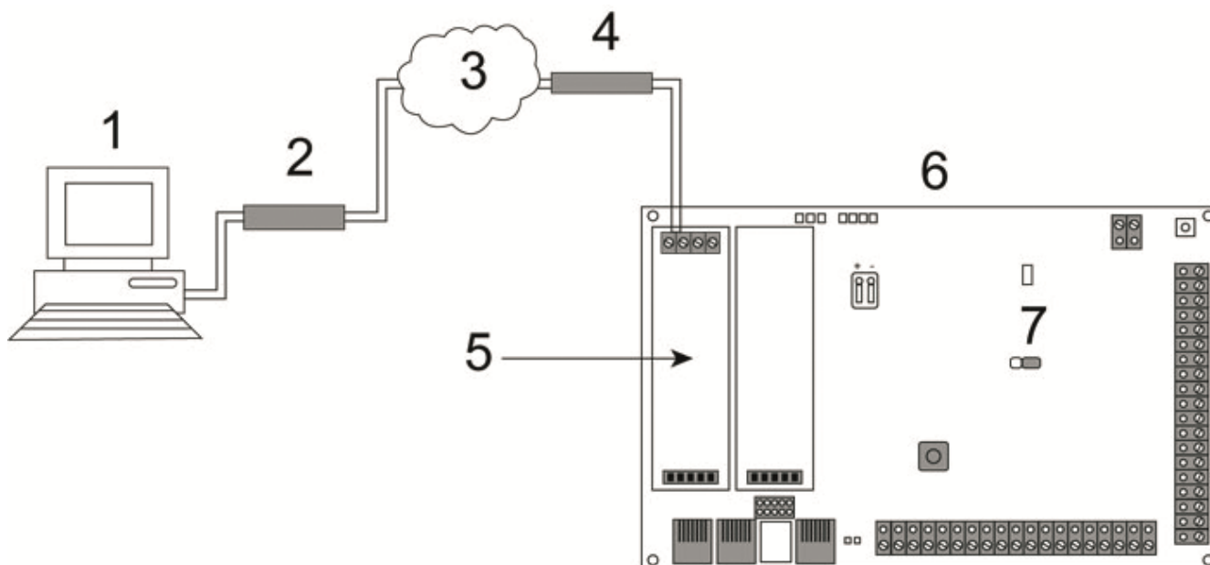
Connexion RTC
